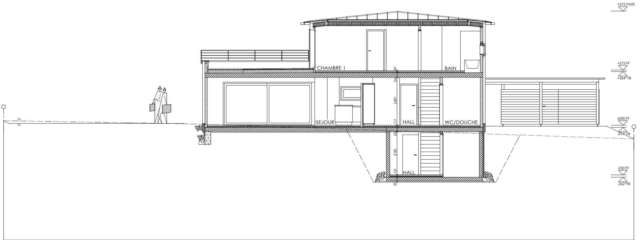
C O U P E A - A
