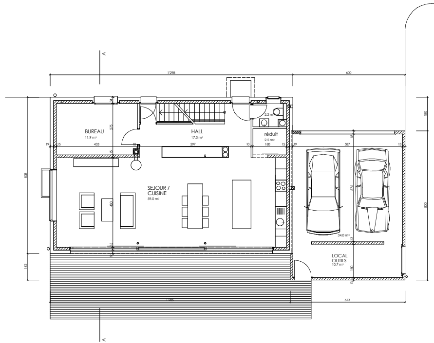
REZ-DE-CHAUSSEE
