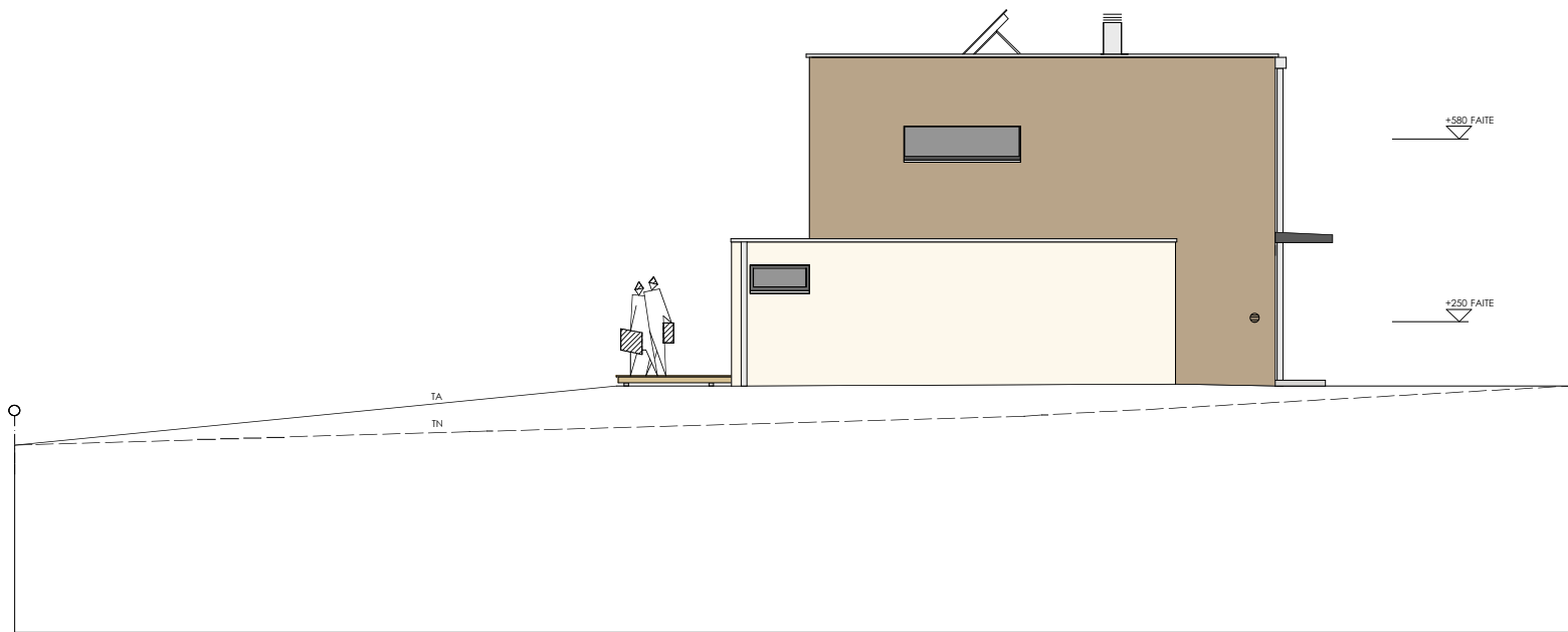
F A C A D E N O R D - E S T
